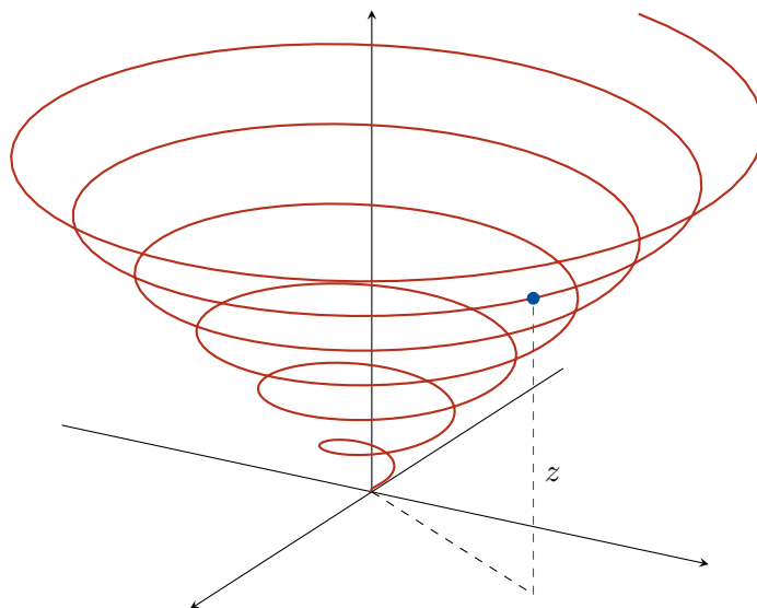
Figur 1: En konisk helix
